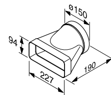
Eindstuk voor platte buis DFKE 215
