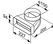
Hoek-adapter voor platte buis DFKA 215
