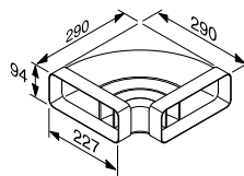
Bochtstuk voor platte buis DFKB 90 H
