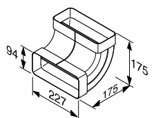
Overgangsstuk voor platte buis DFKB 90 V
