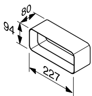
Verbindingsstuk voor platte buis DFKV 289
